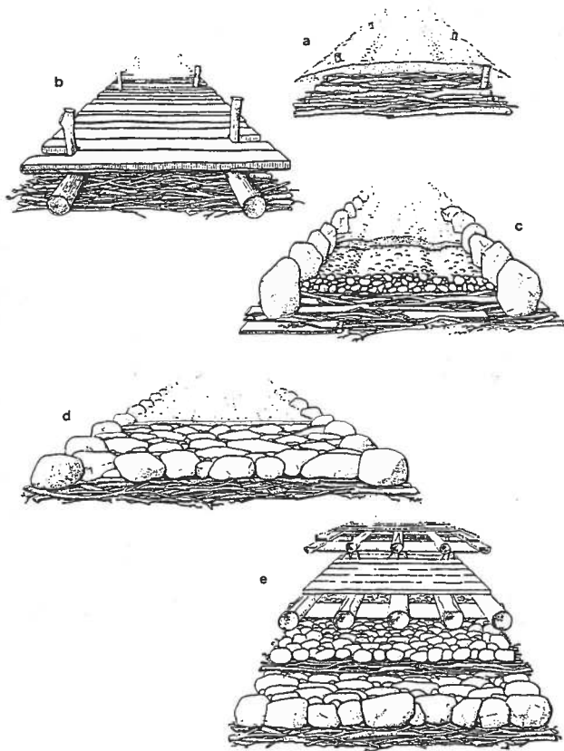
Figur 3. Vejkonstruktioner over blødbundede områder. a: grenvej, Risby, vikingetid c.800; b: plankevej, Speghøje mose, bronzealder c. 1300 f.Kr.; c: stenlagt vej, Risby, vikingetid c.1000; d: stenlagt vej, Broskov c.300; e: vejdæmning, jernalder-vikingetid, Sjellebro. Tegning: Jens Kirkeby; efter Jørgensen 1988.
