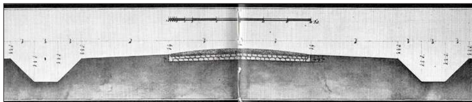
Tværsnit af hovedlandevejen mellem Ringsted og Slagelse. Uden for stenvejen er vist jordveje og yderst i begge sider 3 fod dybe grøfter. Tegning på Rigsarkivet.
